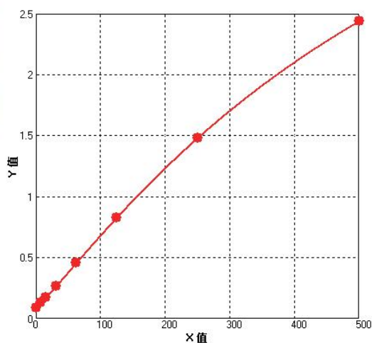
人GM-CSF参考标准曲线
