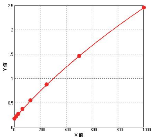
人 IL-6 参考标准曲线
