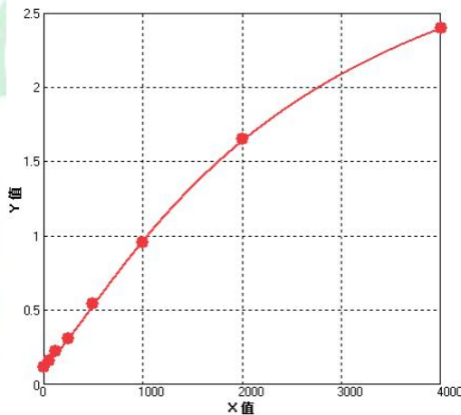
人S100B参考标准曲线
