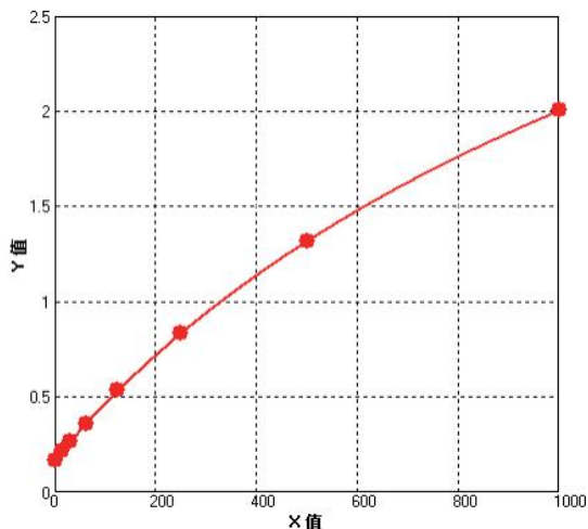
人 TGF- \beta 1 参考标准曲线
