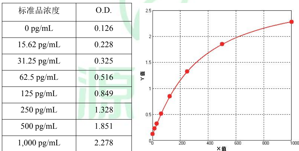
人VEGF参考标准曲线
