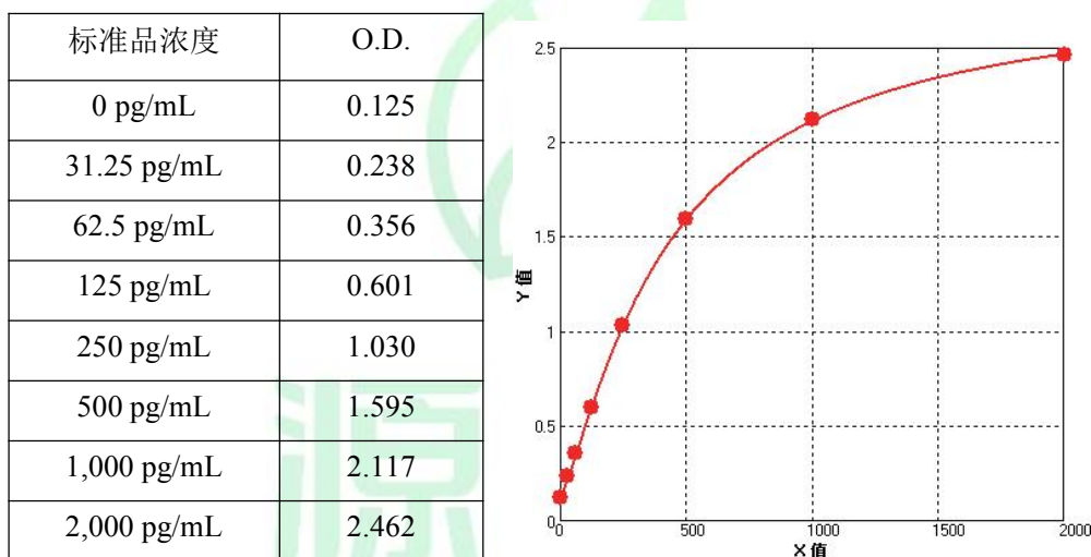
人L-FABP参考标准曲线
