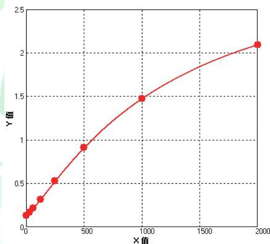
人 COL1A1 参考标准曲线
