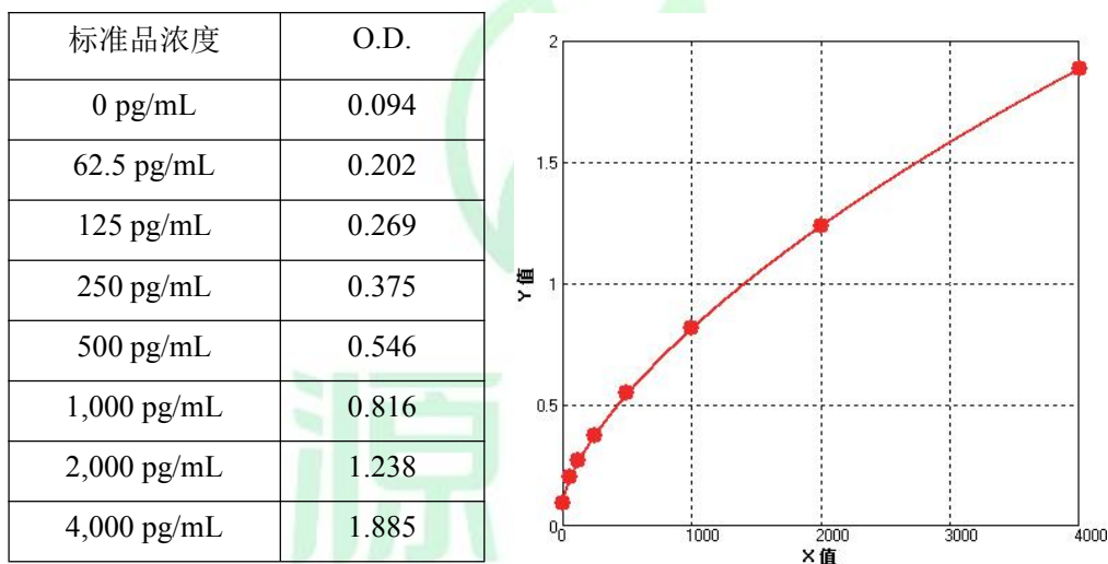
人 CDH3 参考标准曲线
