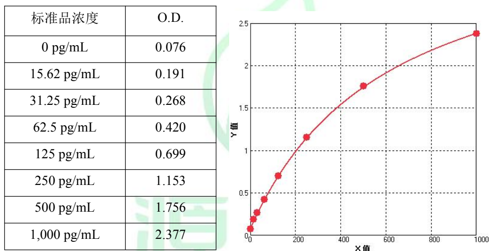
人NKR2B4参考标准曲线
