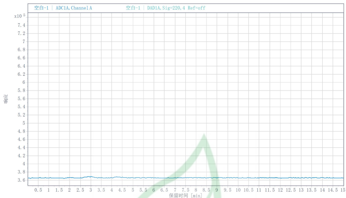
空白谱图
