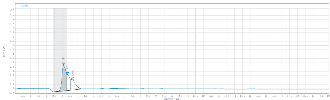
空白谱图
